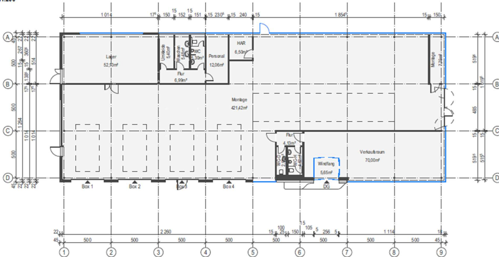
Grundriss EG M1:200
