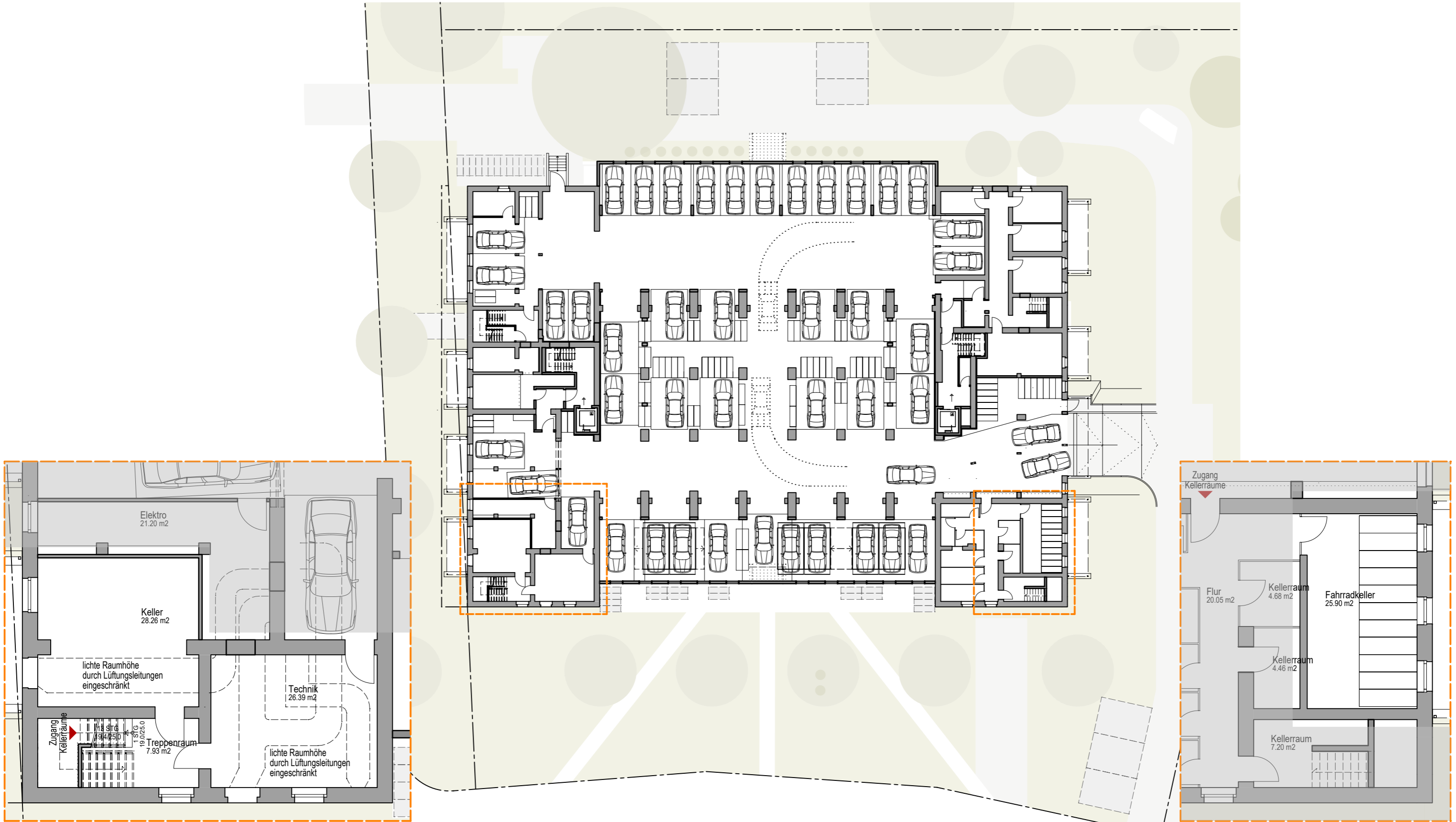
Grundriss Kellerräume, M 1:125 Zugang über internes Treppenhaus
